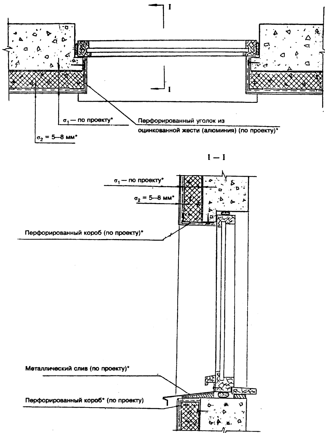
Рисунок А14 — Фрагмент примыкания теплоизоляционного слоя к оконному проему (вариант "с четвертью")
