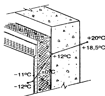
Рисунок 1 — Температурная кривая зимой
