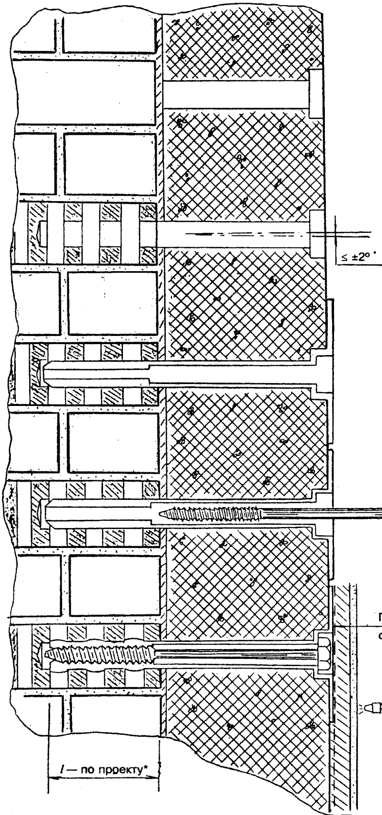
Рисунок А7 — Крепление плиты утеплителя с помощью пластмассовых дюбелей тарельчатого типа с металлическим стержнем (вариант: стеновой материал из пустотелых блоков)
