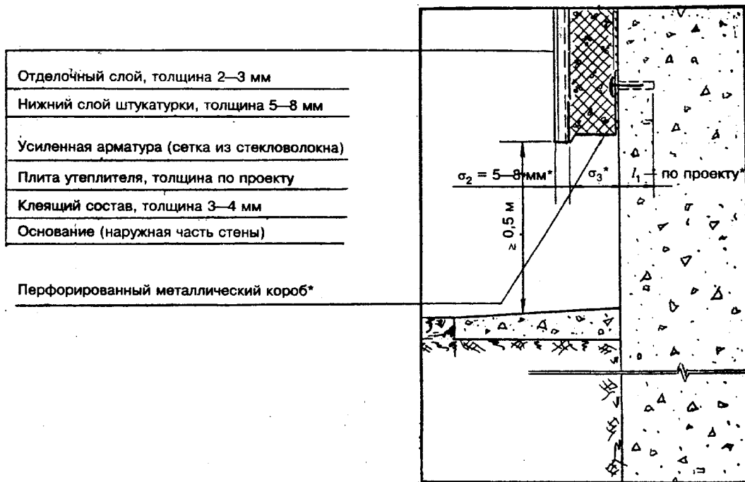
* Контролируемый параметр Рисунок А9 — Крепление теплоизоляционного схода на нижней части стены
