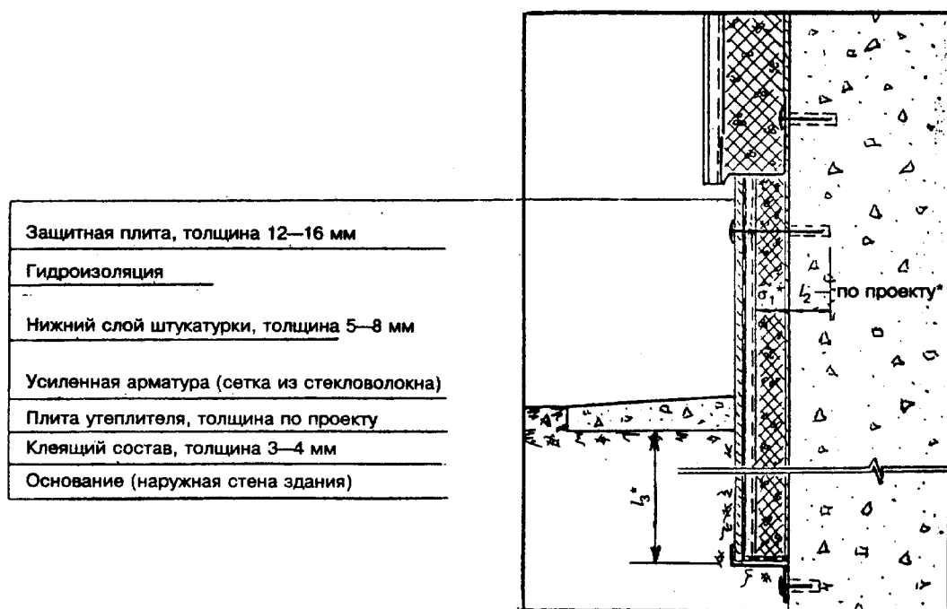
* Контролируемый параметр Рисунок А10 — Фрагмент утепления нижней (и ее заглубленной) части стены здания
